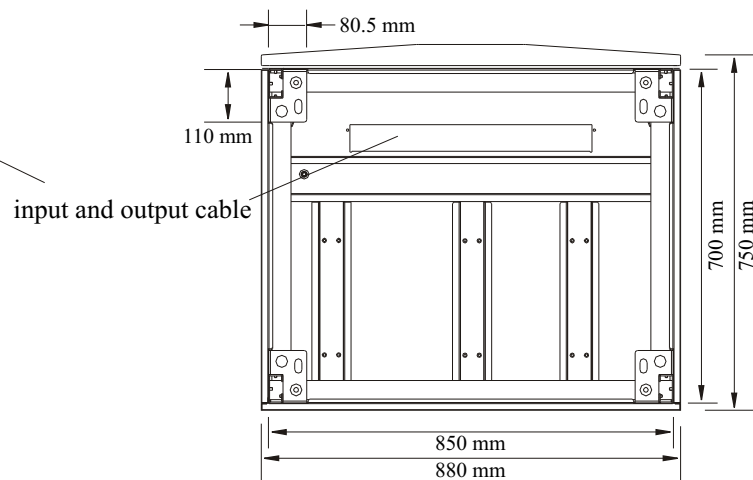
Tampak bawah
