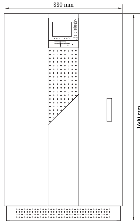
Tampak depan
