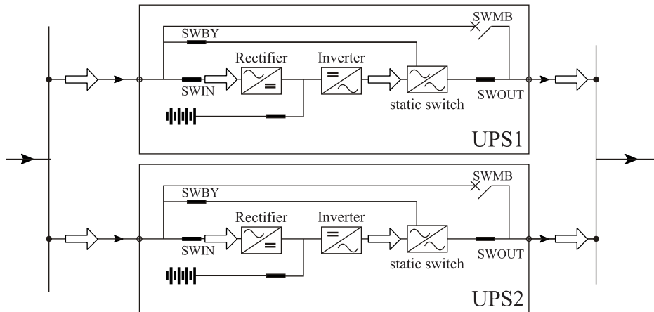
diagram koneksi paralel
